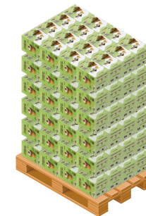
1 x 80x120 cm PALLET Qt. 6 levels (h 182,5 cm) Qt. 120 carton boxes Qt. 4.800 Chocup® Pistàs
